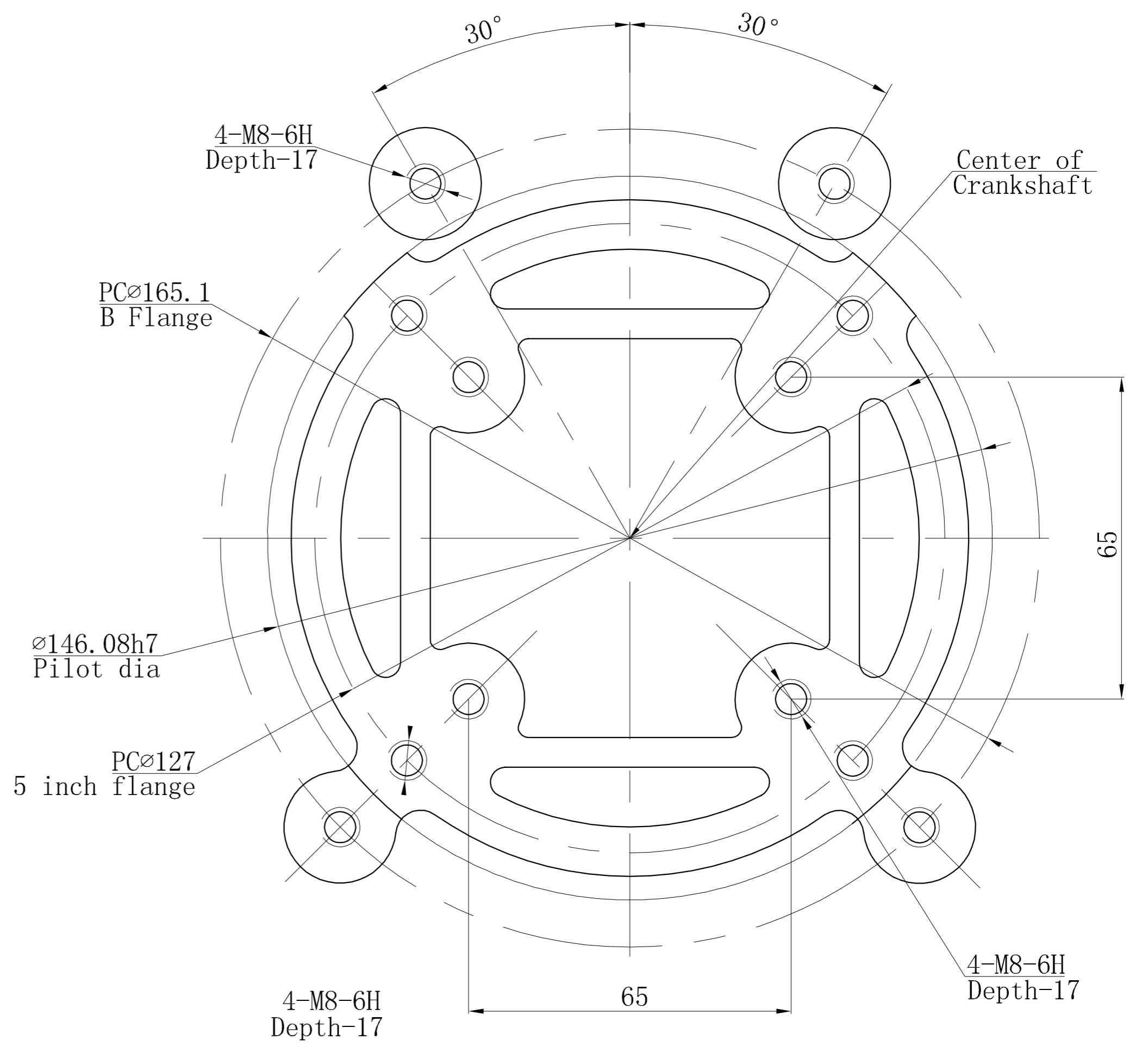
PTO Flange
