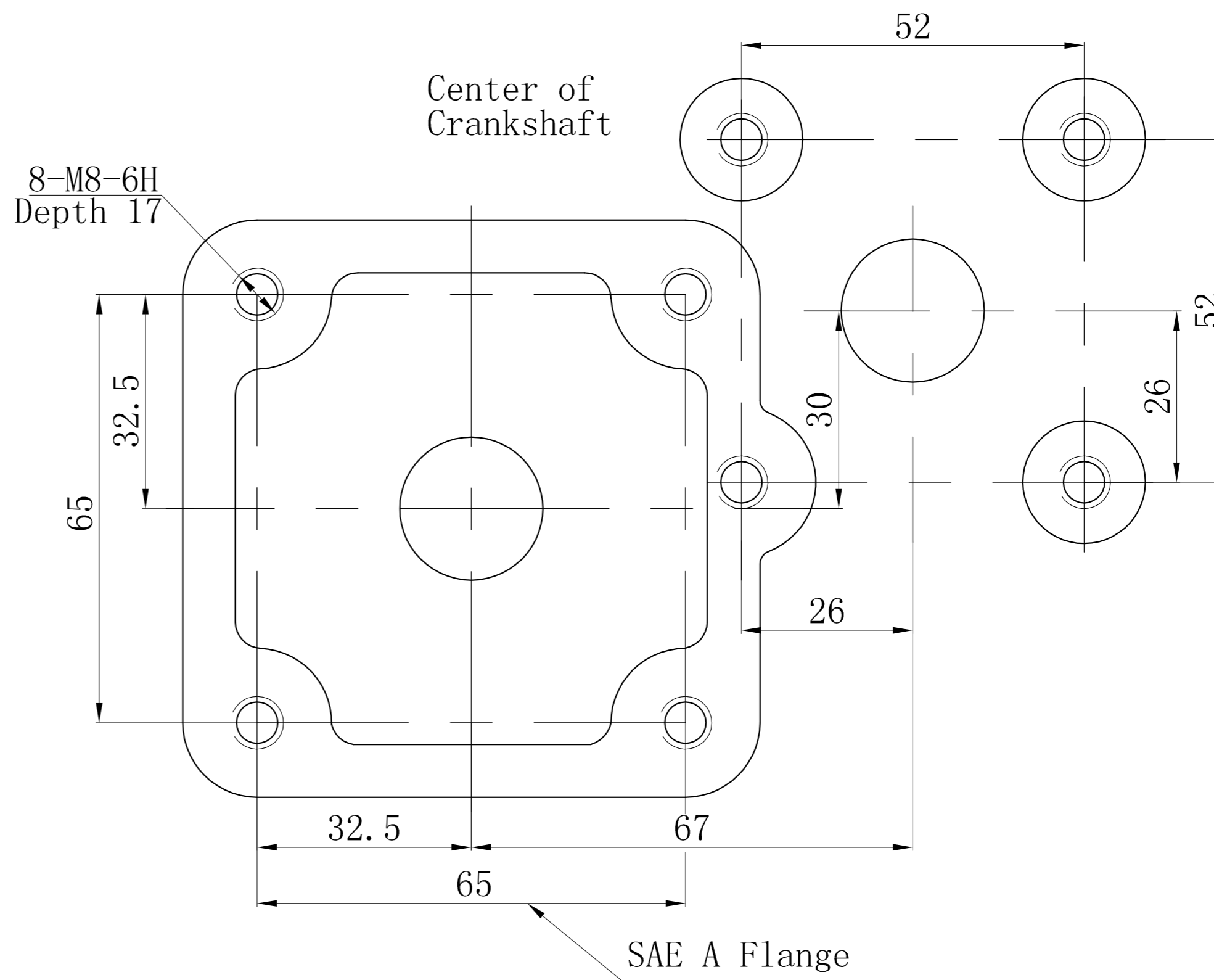
PTO Flange
